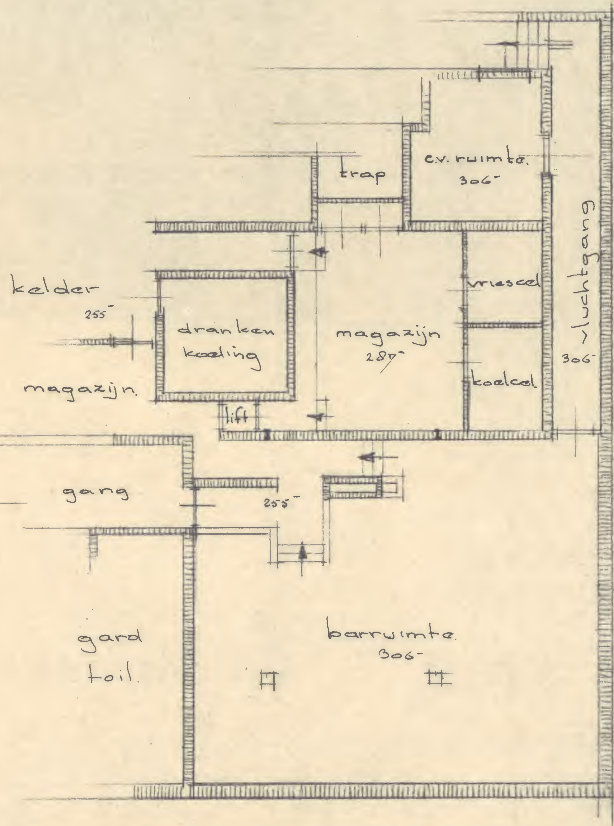
ged. platte grond kelder, bestaand.
